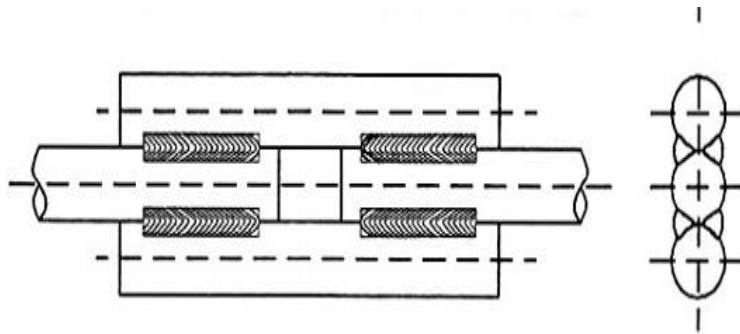
c) Liên kết hàn có sử dụng ốp tấp bằng thép cốt
