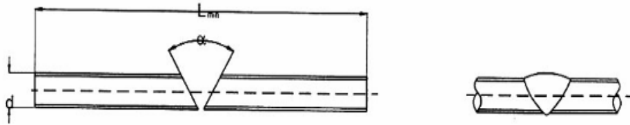
a) Hàn đối đầu, L_{\min} = 8d + 500
