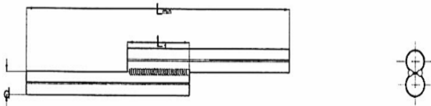
d) Hàn ghép chồng, L_{\min} = 8d + L_1 + 500 .
