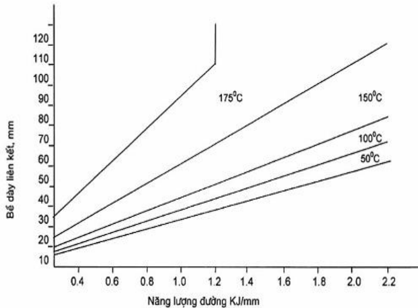
Hình 7 - Đồ thị nung nóng sơ bộ cho các liên kết hàn ốp táp, ghép chồng và đỉnh, áp dụng cho thép cốt có hàm lượng cacbon tương đương không lớn hơn 0,42 %.
