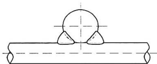
Hình 5 - Liên kết hàn chữ thập
