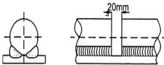
a) Liên kết hàn có sử dụng ốp tấp bằng thép tấm
