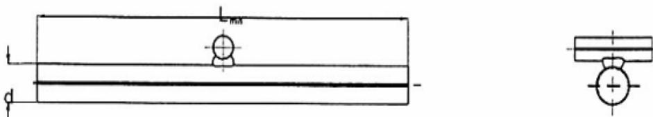
c) Hàn chữ thập, L_{\min} = 8d + 500
