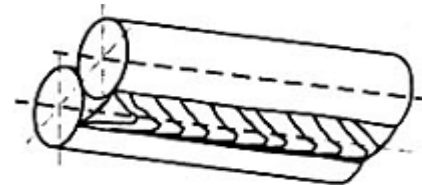
d) Hàn ngửa (trục hàn nằm ngang, chiều dày mối hàn thẳng đứng)
