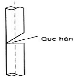
b) Vị trí hàn ngang (thép cốt thẳng đứng);
