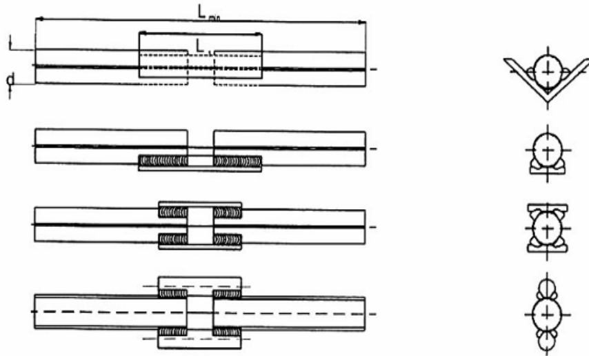
b) Hàn ố tấp, L_{\min} = 8d + L_1 + 500
