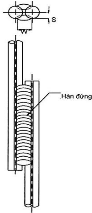
Hình 3 - Liên kết hàn ghép chồng
