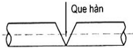
a) Vị trí hàn bằng (thép cốt nằm ngang; vát mép hai đầu; góc vát mở phía trên);
